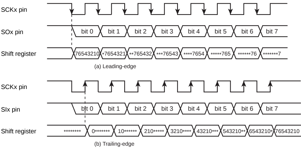
Figure 11-17 Shift Edge
