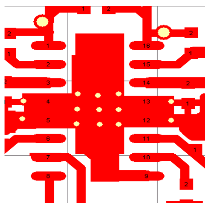
TOP (16 Ld SO)
