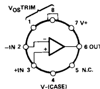
TO-99 (J-Suffix)
