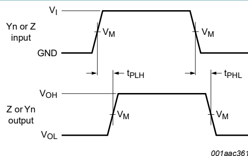
Fig. 13. Input (Yn or Z) to output (Z or Yn) propagation delays
