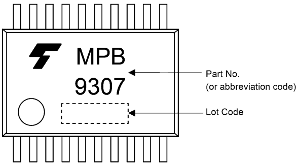
Fig. 6.2 TSSOP20
