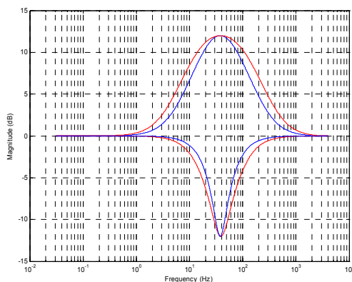
Figure 69 EQ Band 2 – EQ2BW=0, EQ2BW=1
