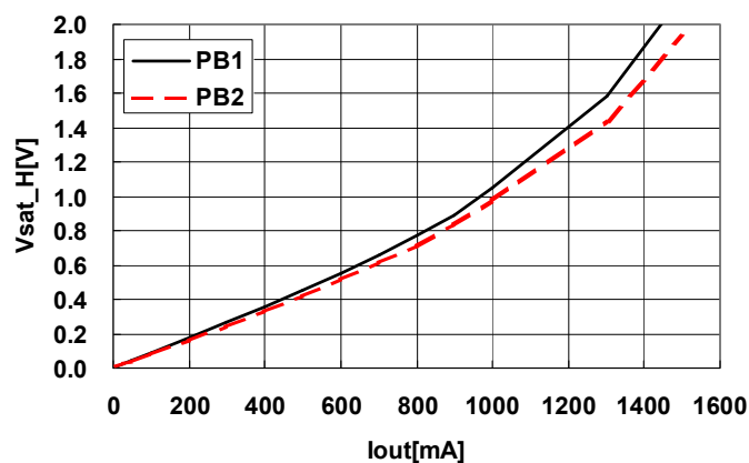
Iout VS. Vout VDD=5V T_a=25[^\circ\text{C}]
