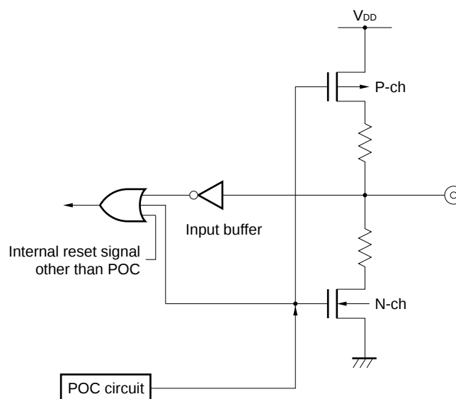
(6) \overline{RESET}
