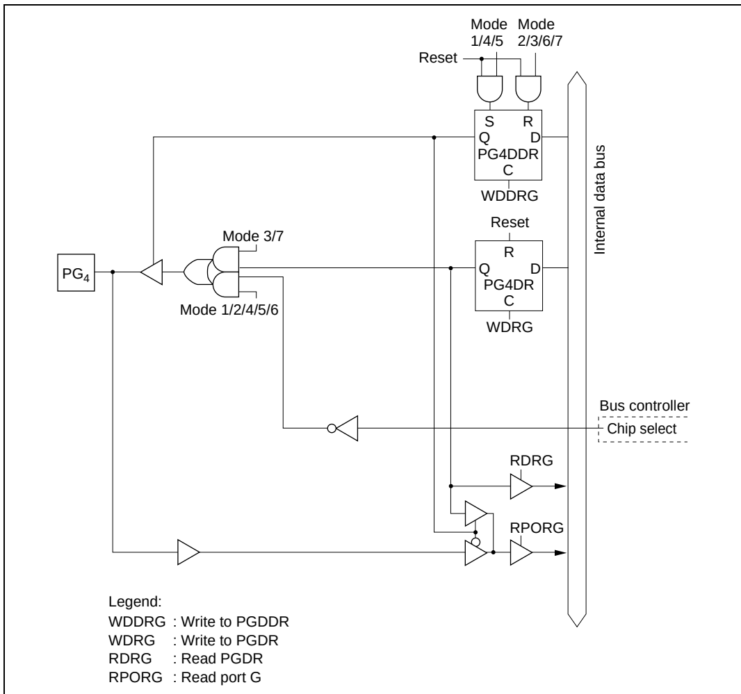
Figure C.11 (d) Port G Block Diagram (Pin PG 4 )
