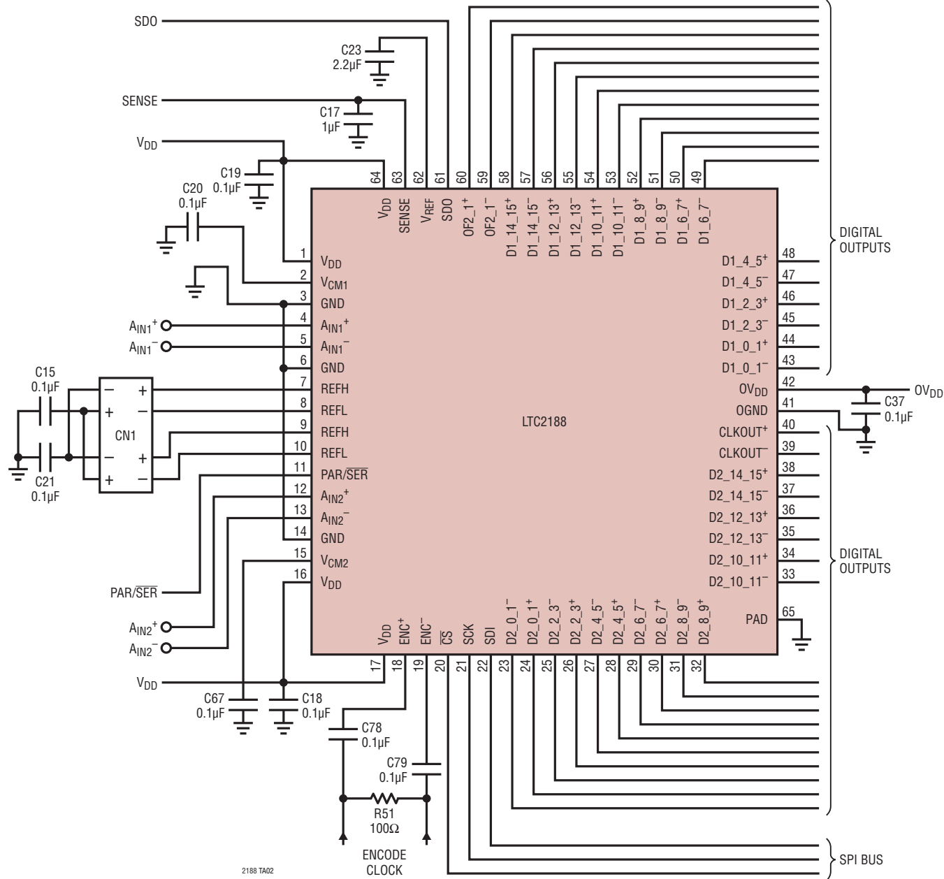
LTC2188 Schematic
