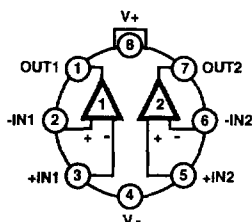
HA-5142 (METAL CAN)
