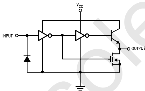
1/4 MM78C29/MM88C29
