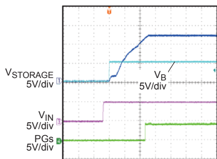
V_{STORAGE} Charge
