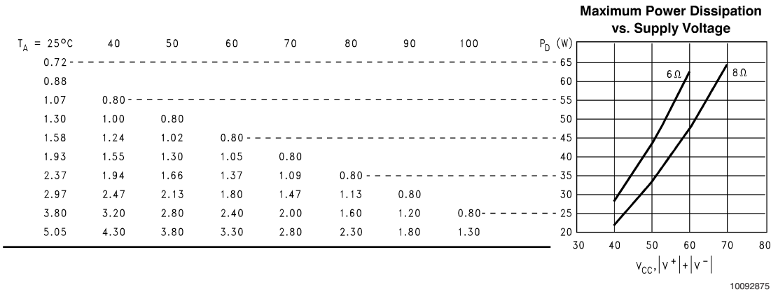
Max Heatsink Thermal Resistance (°C/W) at the Specified Ambient Temperature (°C)
