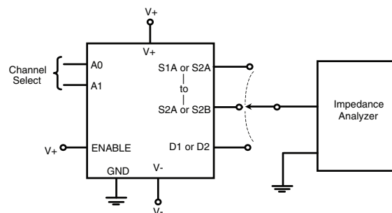
Fig. 8 - Source/Drain Capacitance
