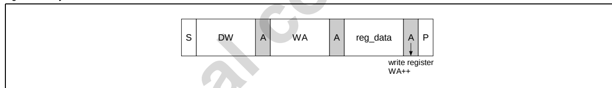
Figure 25. Byte Write
