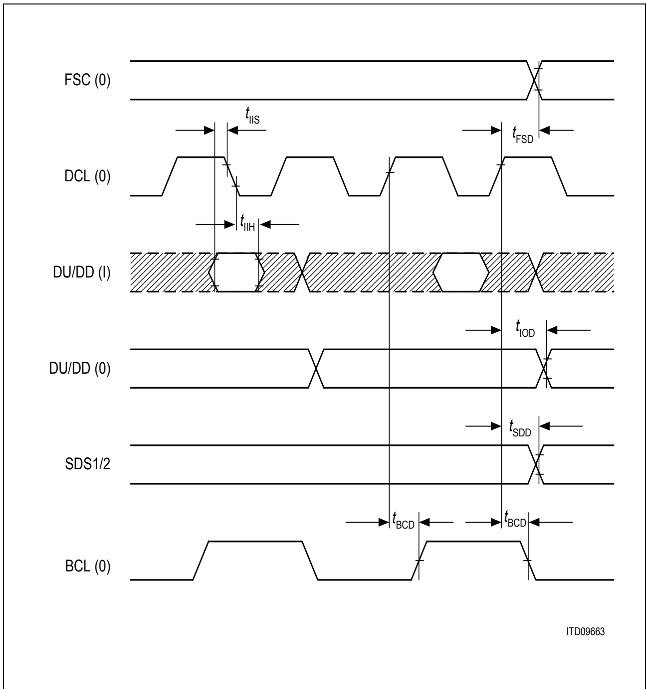
Figure 79 IOM ® Timing
