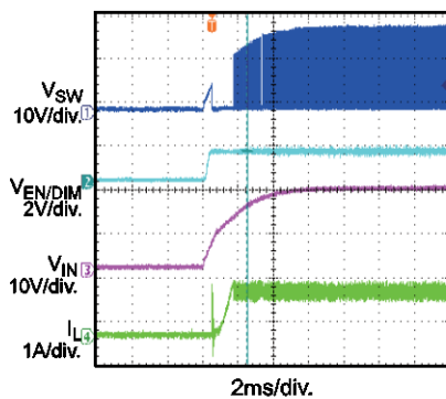
VIN Start-Up
