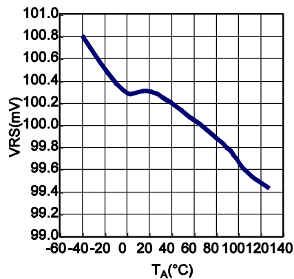
VRS
