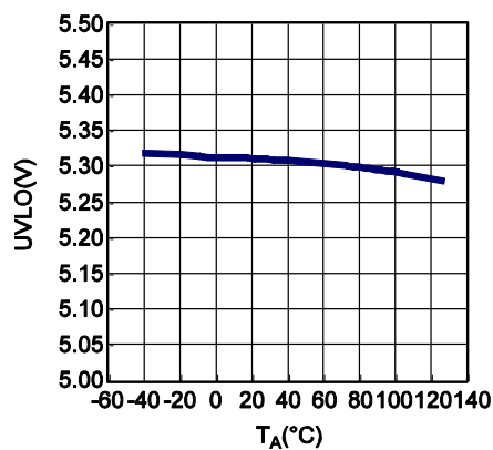
VIN UVLO
