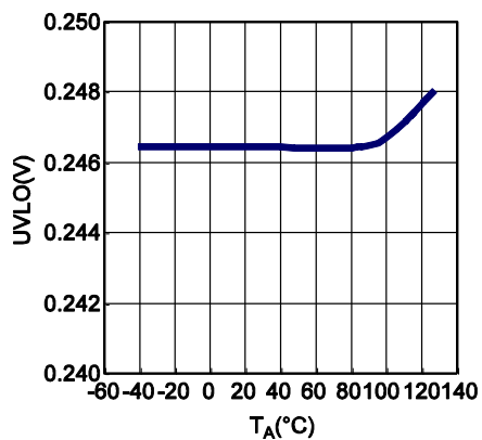
EN UVLO
