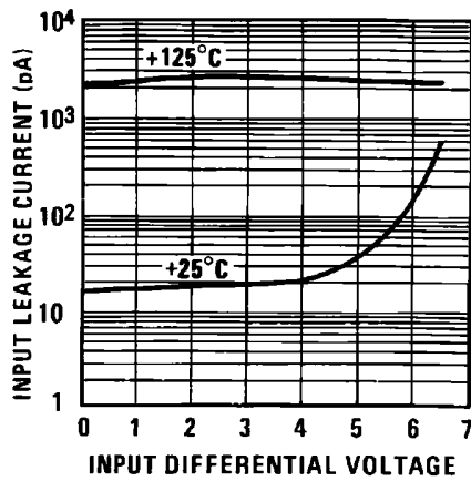
Input Leakage
