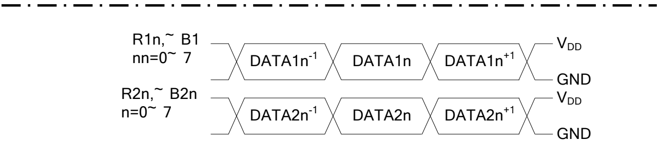
LVC MOS Data Input
