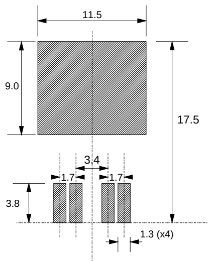
Fig.34. SOT426
