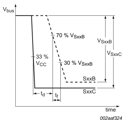
Fig 4. Timing parameters
