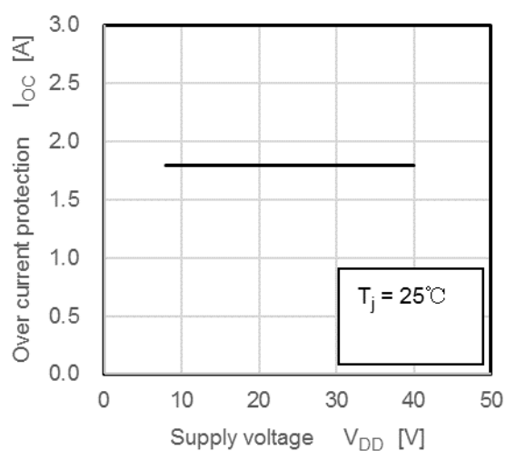
I_{OC} - V_{DD}
