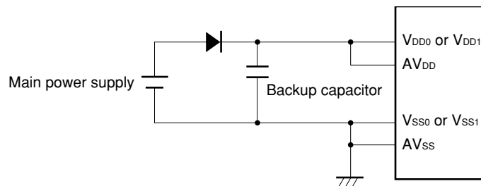
Figure 13-21. Processing of AV DD Pin
