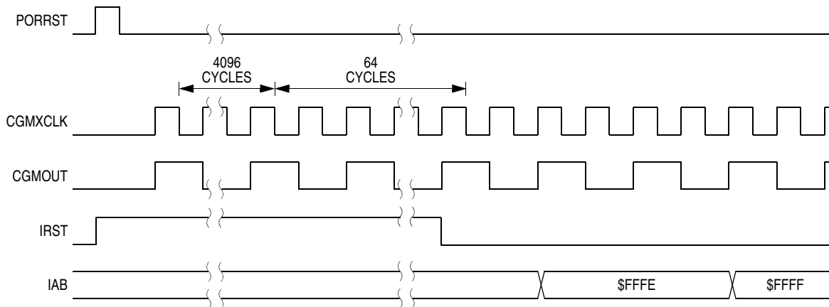
Figure 13-6. POR Recovery
