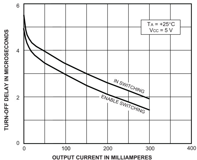
Dwg. GP-066
