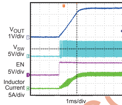
Enable Startup
