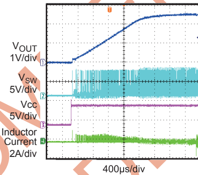
Vcc Startup
