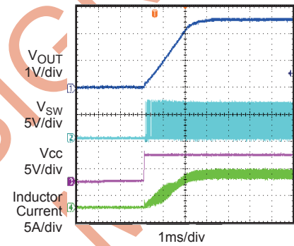
Vcc Startup
