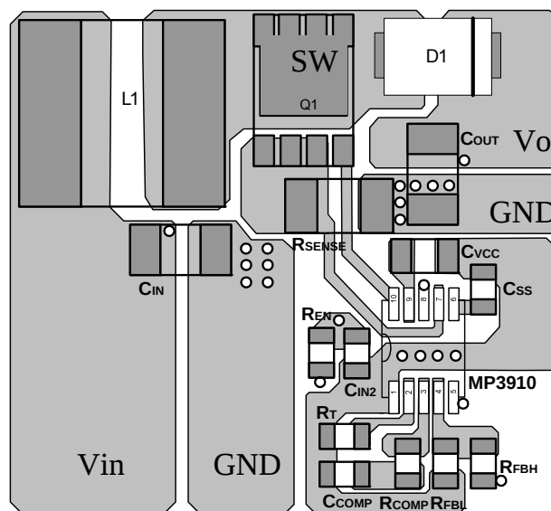
Top Layer
