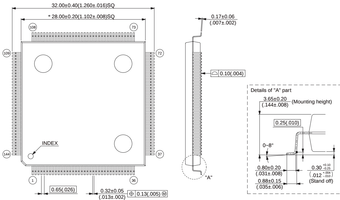
144-pin plastic QFP (FPT-144P-M01)
