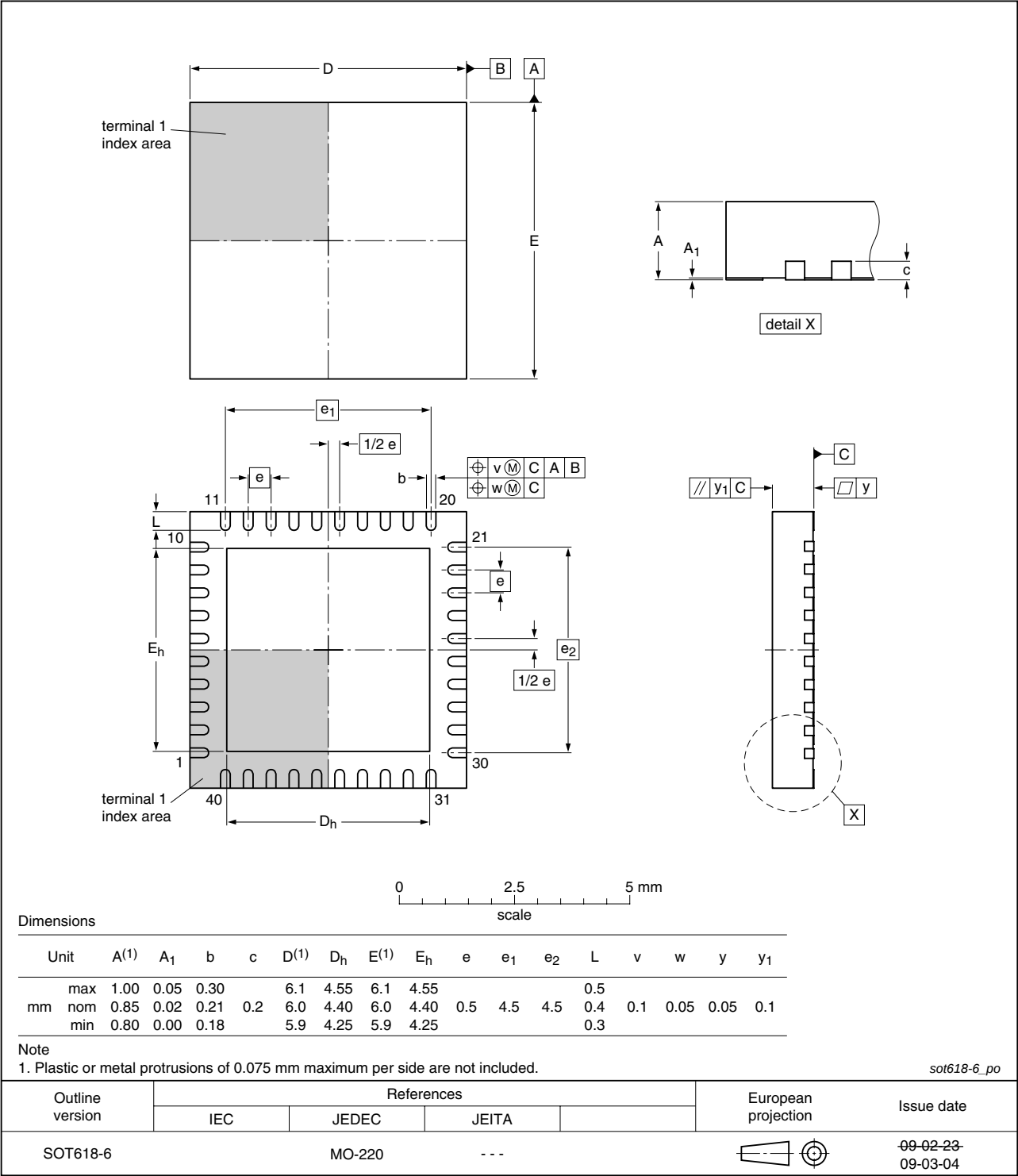
Fig 25. Package outline SOT618-6 (HVQFN40)
