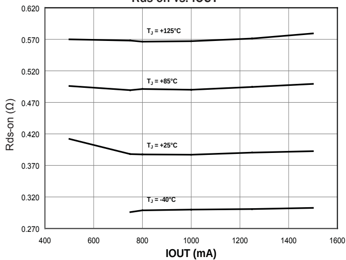
R ds-on vs. IO UT
