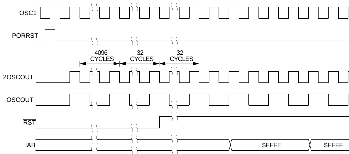
Figure 7-7. POR Recovery
