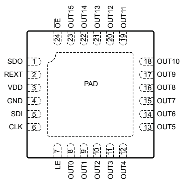
ES Package
