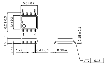
SOP8
