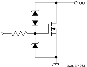
Dwg. EP-063
