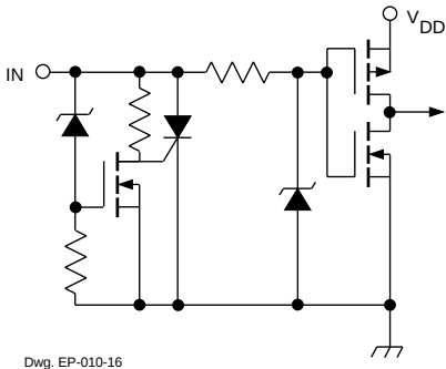
Dwg. EP-010-16
