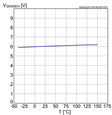
Figure 33. V_{\text{SENSEH}} vs. T_{\text{case}}
