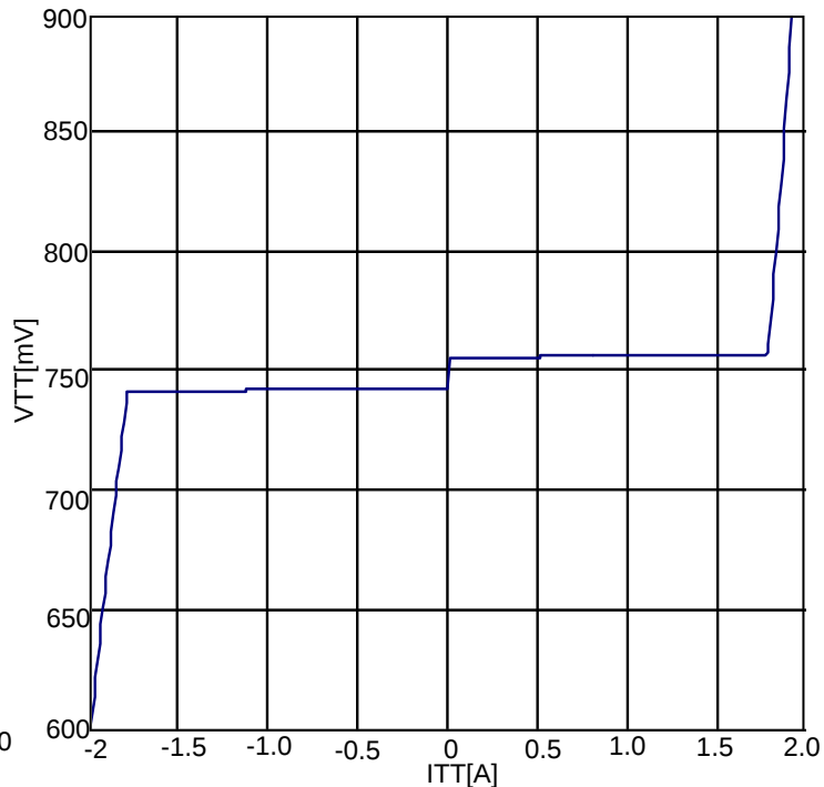
Figure.12 ITT-VTT(DDR3)
