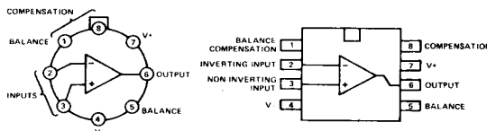
TO-99
