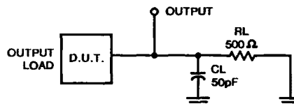
Fig. 4 - Test circuit.
