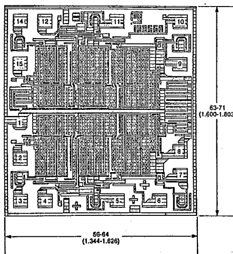
CD4050BH
