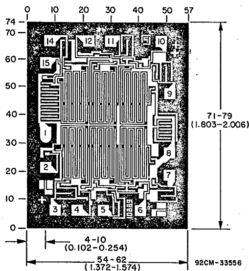
CD4049UBH
