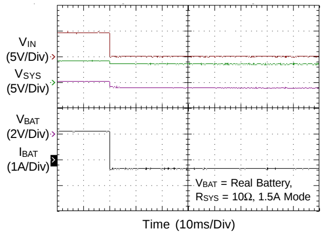
VIN Removal
