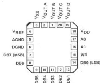
PM-7226HPC 20-PIN PLCC (PC-Suffix)
