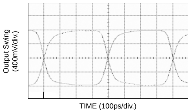
1.25GHz Output (Q – I/Q)
