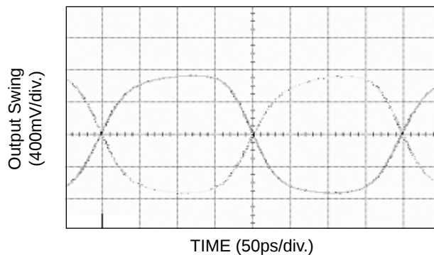
2.5GHz Output (Q – I/Q)
