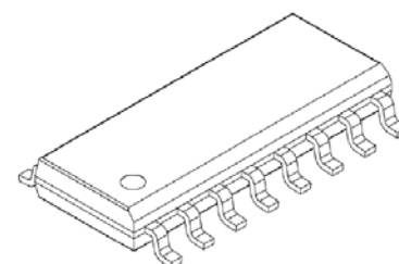
P-SOP16-0410-1.27-002
