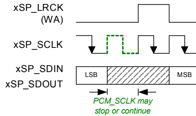
Figure 28. PCM Format—Mode 0
