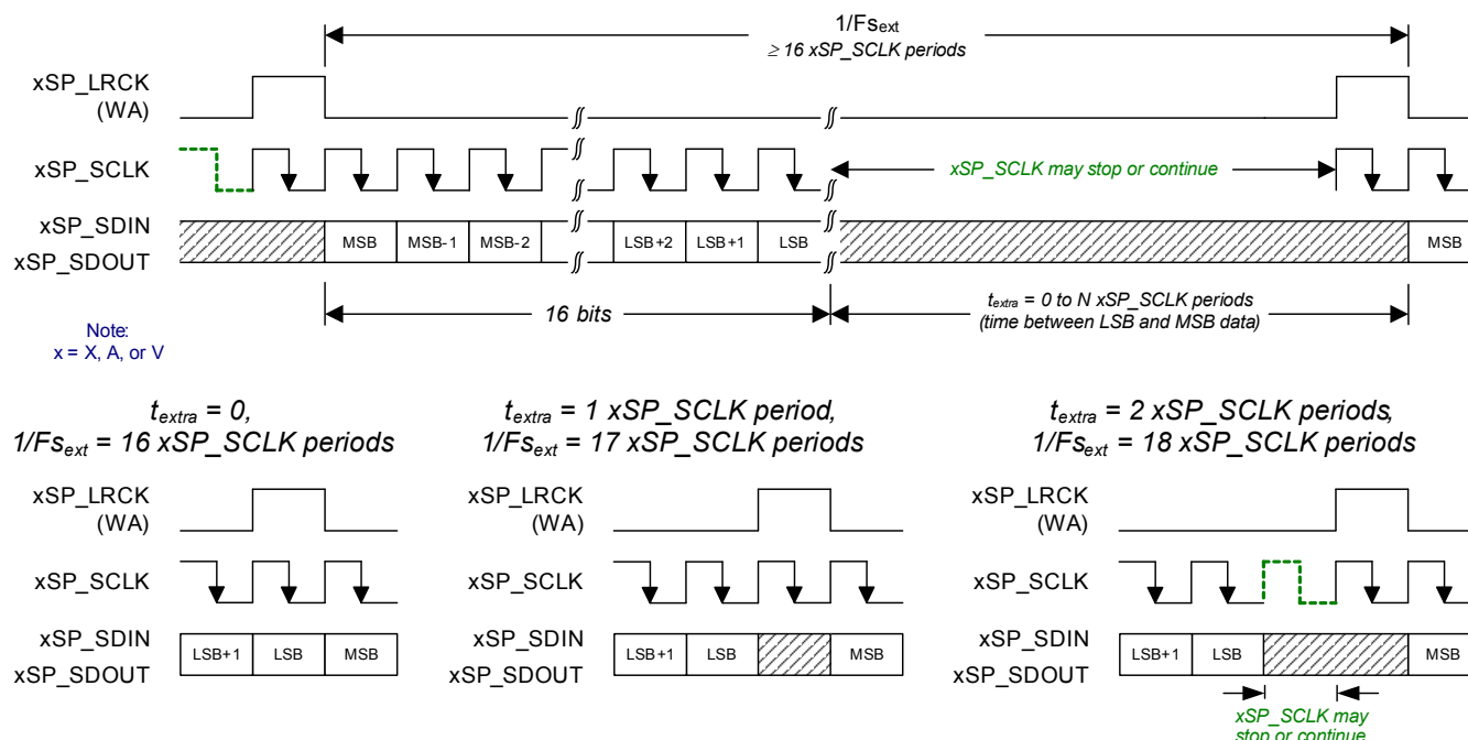
Figure 30. PCM Format—Mode 2
