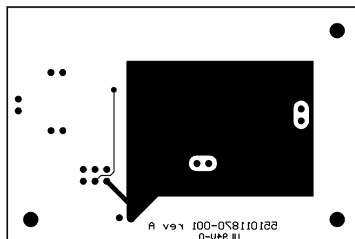
Bottom Layer
