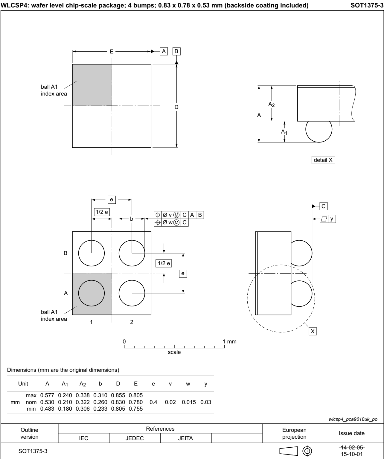
Fig 16. Package outline PCA9618UK (WLCSP4)
