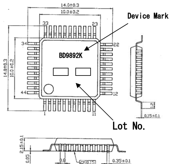
QFP44 (unit:mm)
